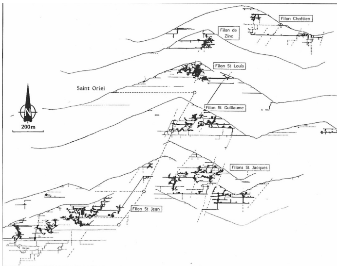
Comparatif entre les différents filons du Neuenberg (vue en coupe nord-sud). Le filon Saint-Louis est de loin le plus excavé...
