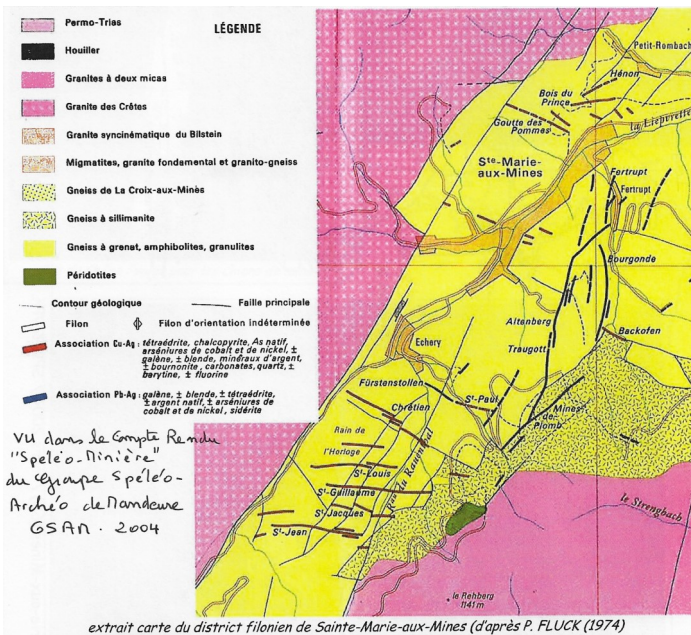
extrait carte du district filonien de Sainte-Marie-aux-Mines (d'après P. FLUCK (1974))
